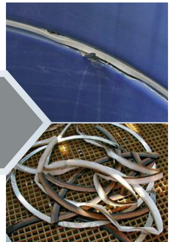
Herkömmliche Hüllringdichtungen
